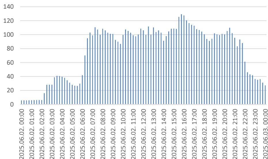
3. ábra Napi villamos teljesítményfelvétel (kW)
